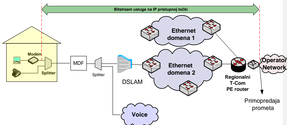
Slika 16. Veleprodajni širokopojsni pristup za pružanje VoIP usluge na IP razini u slučaju kada krajnji korisnik ostvaruje Osnovni pristup mreži putem usluge HT-a
