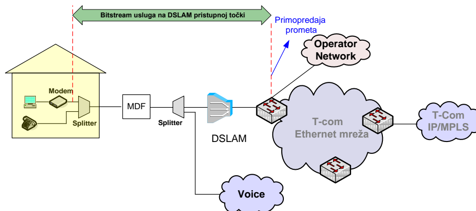
Slika 7. Veleprodajni širokopojsni pristup za pružanje Internet usluge na DSLAM razini u slučaju kada krajnji korisnik ostvaruje Osnovni pristup mreži putem usluge HT-a
