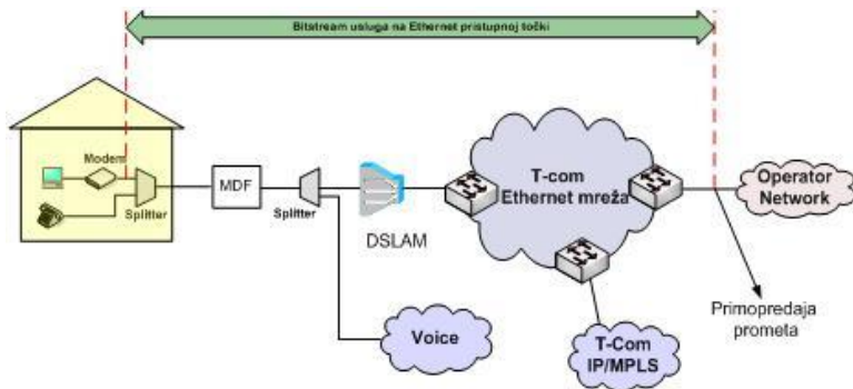
Slika 3. Veleprodajni širokopojasni pristup za pružanje Internet usluge na Ethernet razini u slučaju kada Krajnji korisnik ostvaruje Osnovni pristup mreži putem usluge HT-a.
